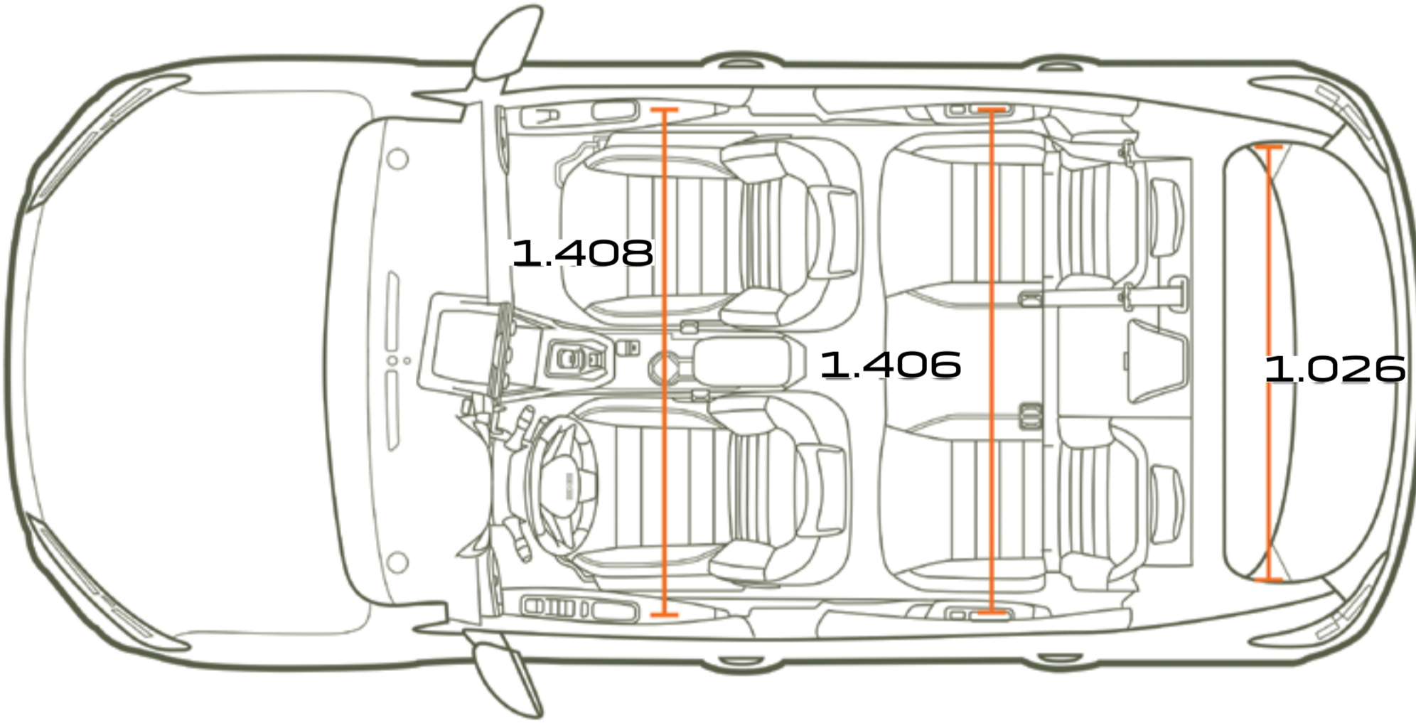
ÜSTTEN GÖRÜNÜM
