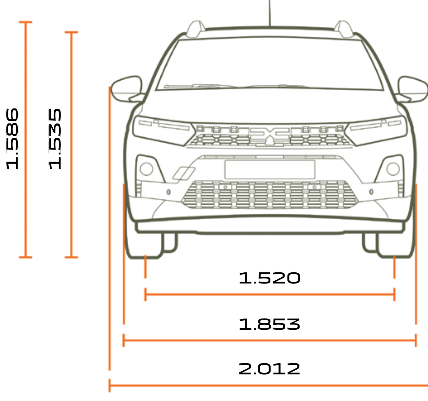
ÖN GÖRÜNÜM
