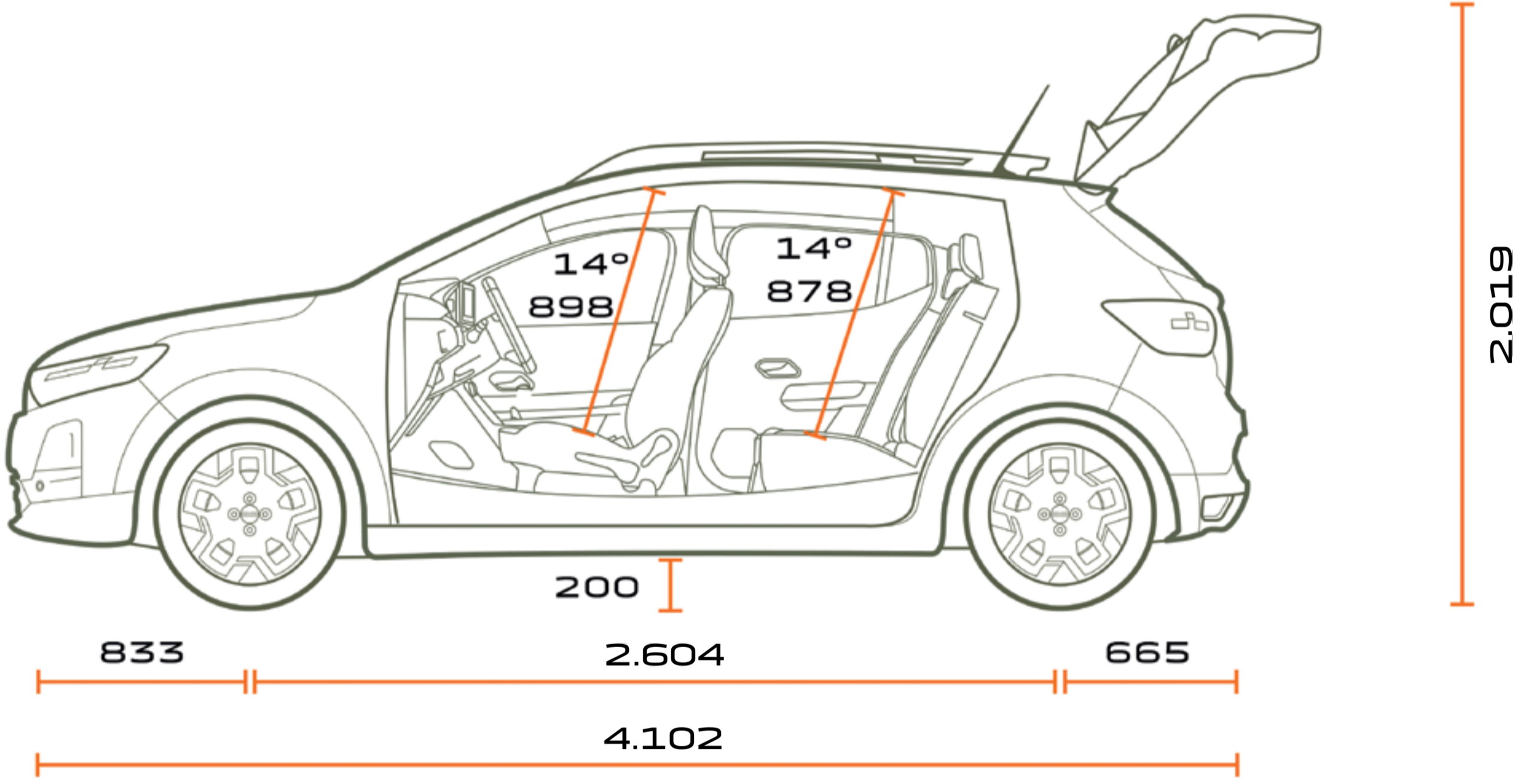
YAN GÖRÜNÜM
